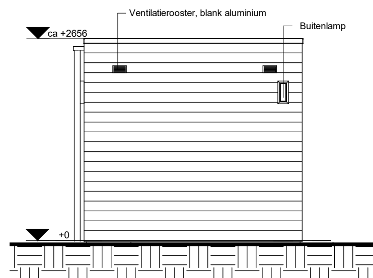
langsgevel achter Schaal: 1 : 50
