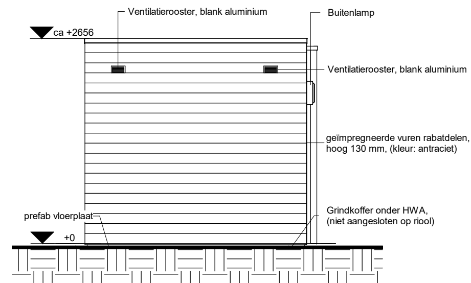
langsgevel tuin/parkeerzijde Schaal: 1 : 50
