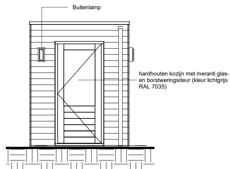
kopgevel rechts Schaal: 1 : 50
